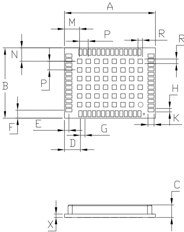
图 2-2 UMD980 机械图
