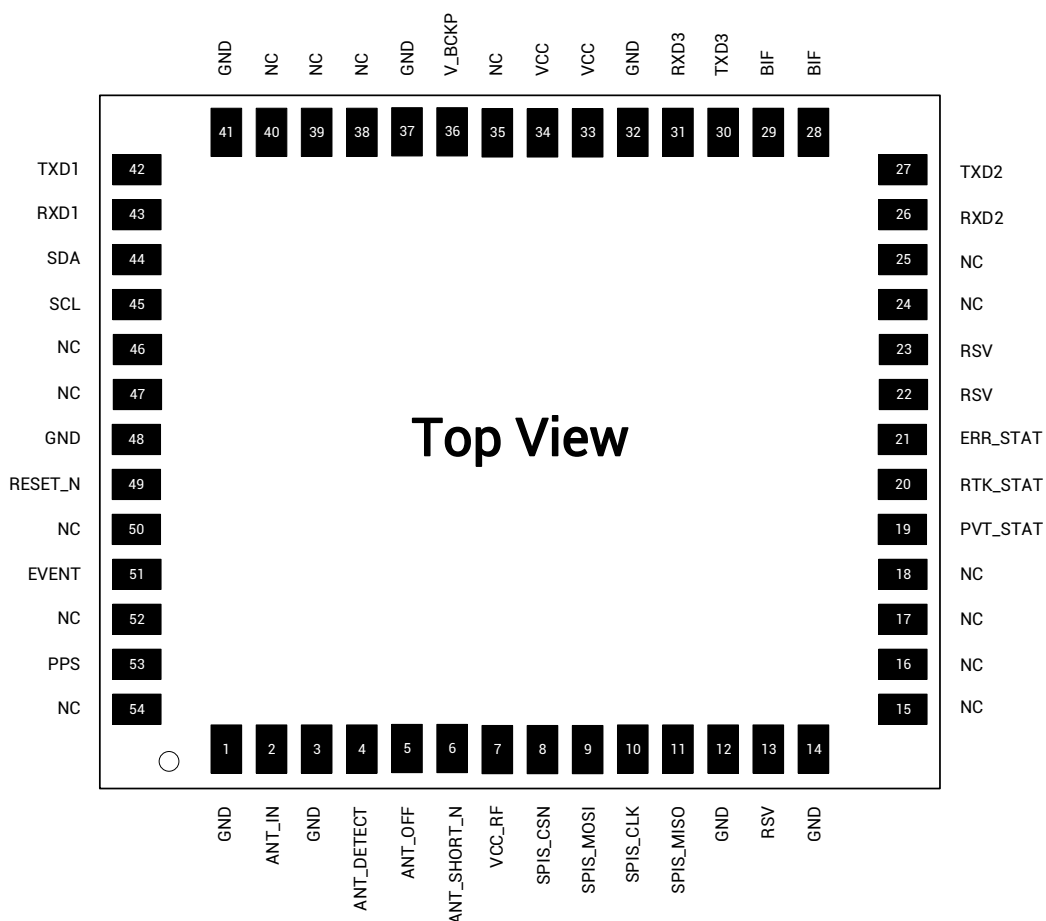
图 2-1 UMD980 管脚图
