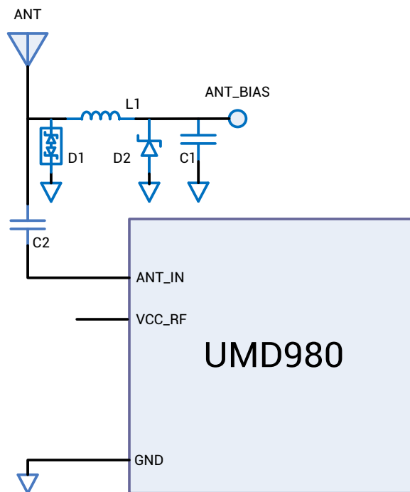
图 3-2 UMD980 外部天线馈电参考电路
