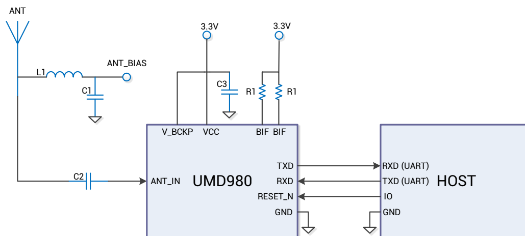
图 3-1 UMD980 最小系统推荐设计
