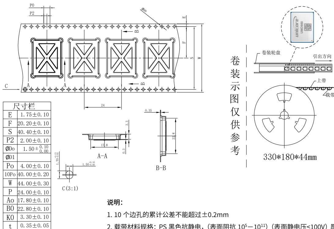
图 5-2 UMD980 模块包装示意
