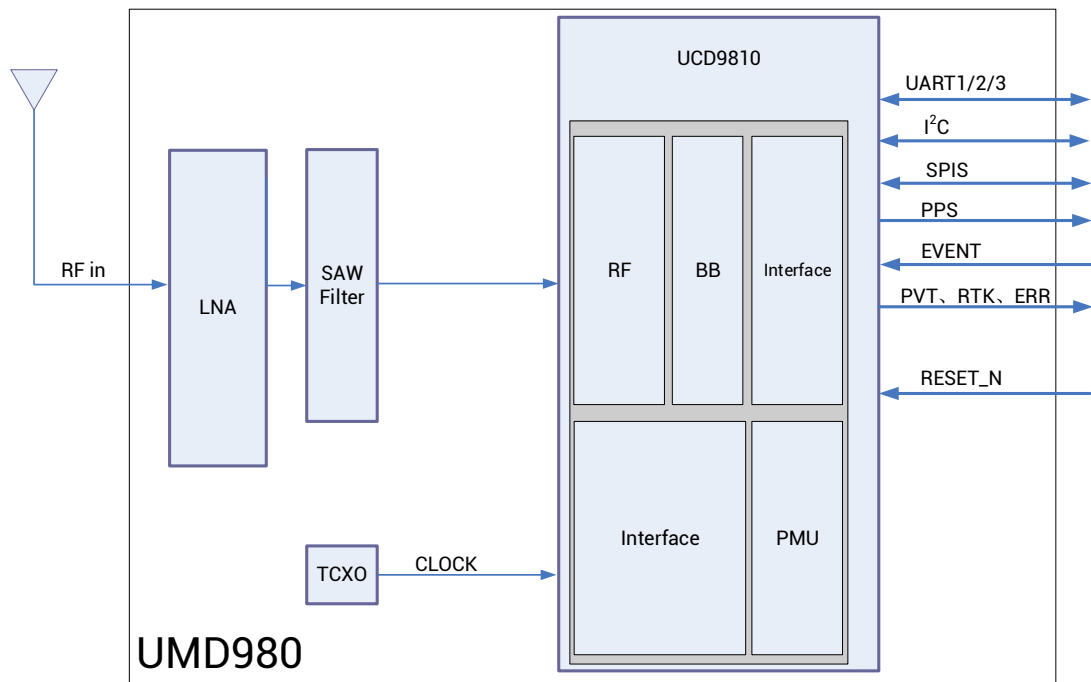
图 1-2 UMD980 结构框图
