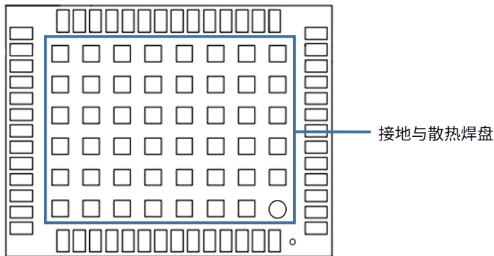
图 3-3 UMD980 接地与散热焊盘（底视图）
